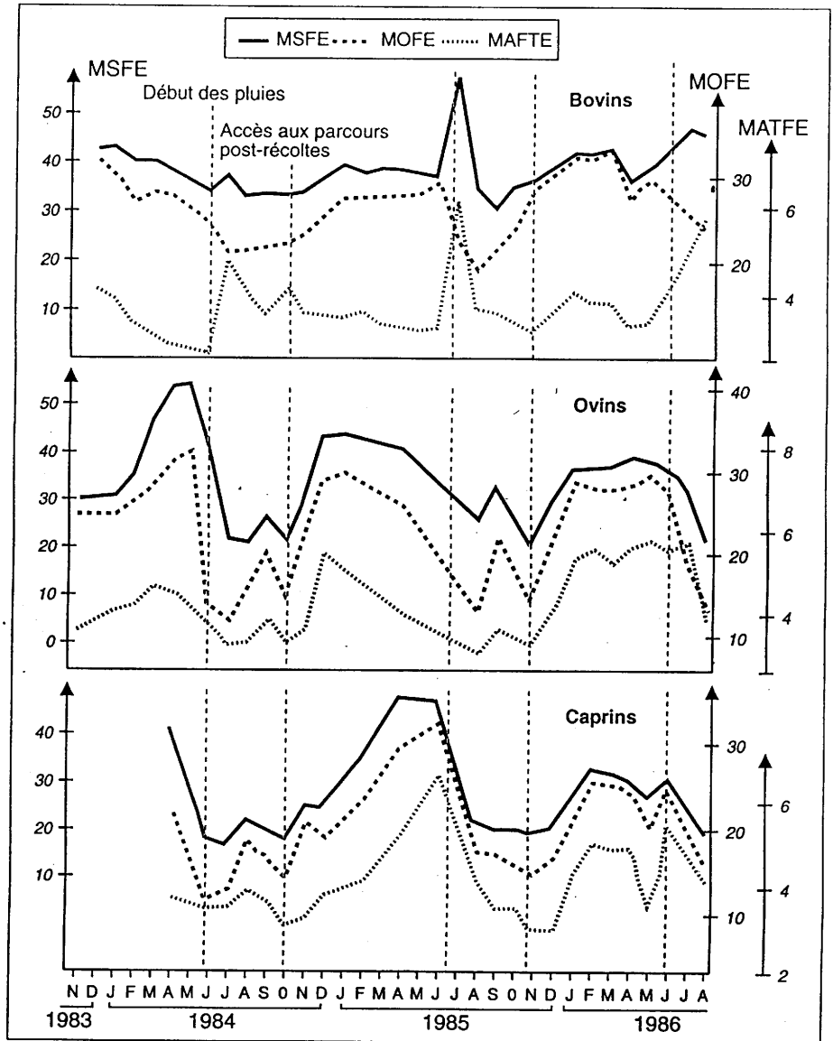
Figure 4. Évolution des quantités (en g/kg P 0.75 ) de matière sèche (MSFE : courbe supérieure), de matière organique (MOFE : courbe intermédiaire) et de matières azotées (MATFE : courbe inférieure) excrétées dans les fèces des ruminants en milieu agro-pastoral au Sine-Saloum (Thyssé-Kaymor, département de Nioro-du-Rip, Sénégal) [6].
